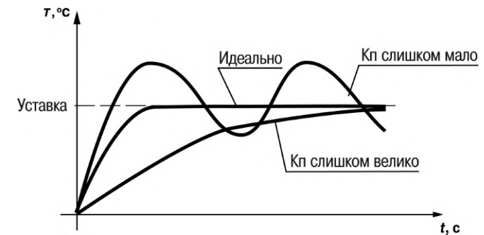
Рисунок 10.21 – Влияние K п на выход на уставку
