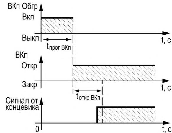
Рисунок 10.2 – Работа воздушного клапана
